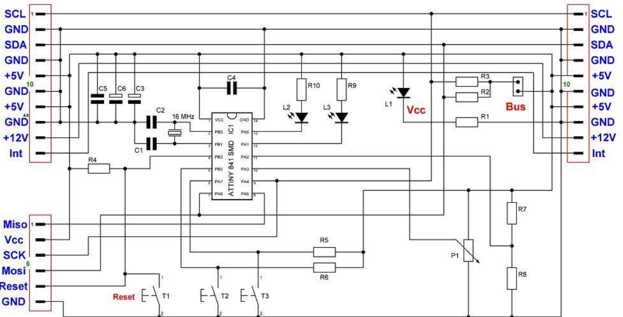
Schaltung P173 mit Attiny 841 und Quarz, 2 Taster, 2 LEDs, Poti
