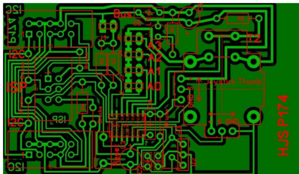
Platine P174 in der Durchsicht
