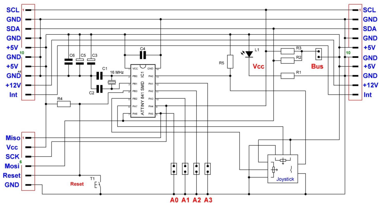
Schaltung P174 mit Attiny 841 mit Quarz, Joystick und Adresswahl
